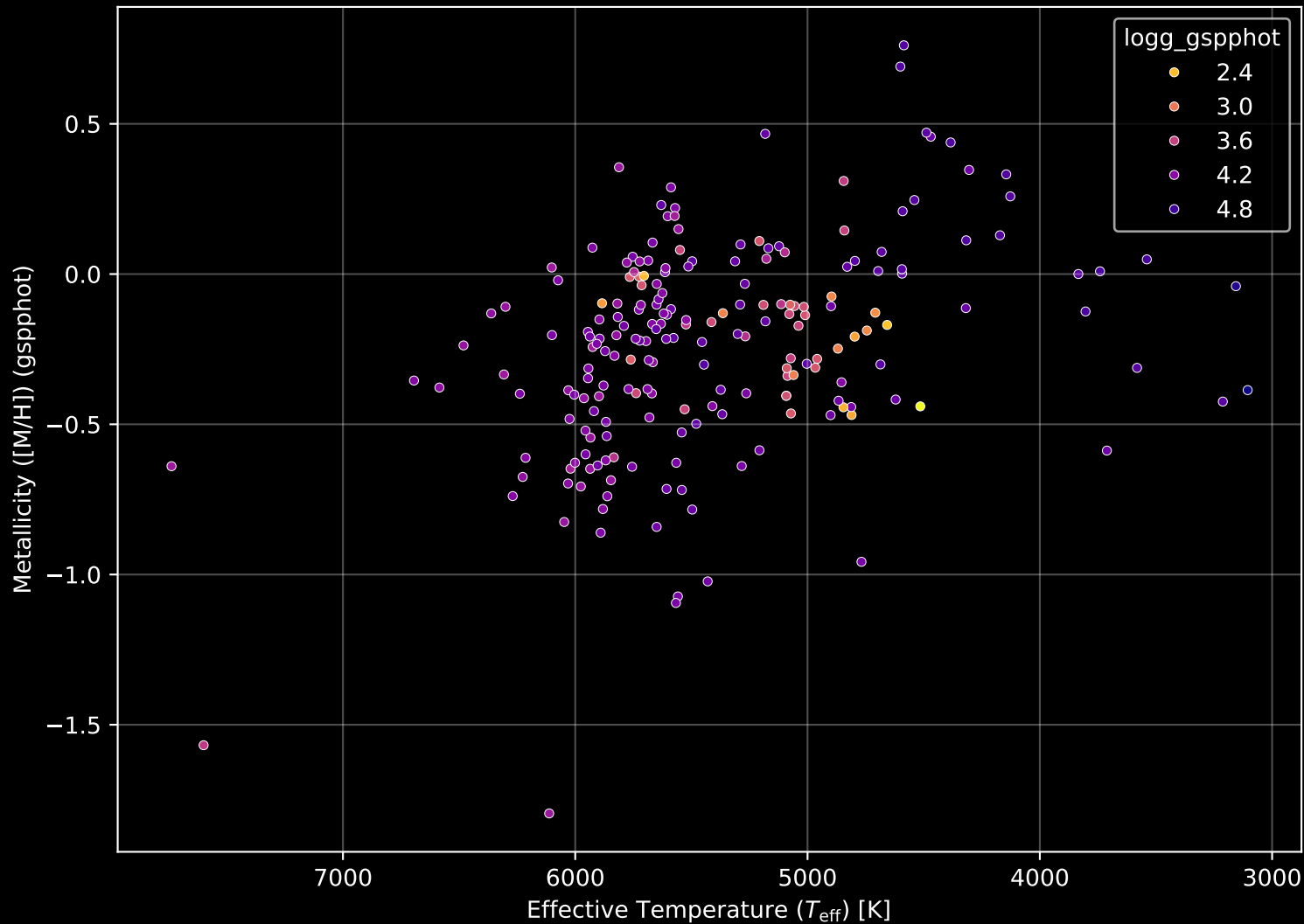
APOGEE DR17 Field: [101+89_MGA] Stellar Population Parameters (n= 206)
